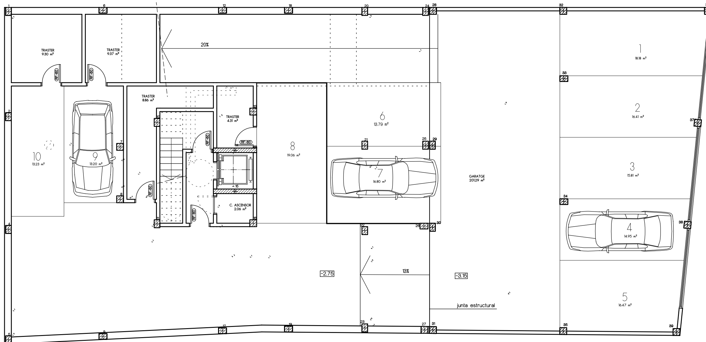
PLANTA SOTERRANI SUP. CONSTRUIDA SOTERRANI 437.34m2
